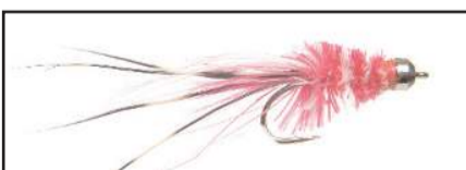
SilungaKrafla bleik
