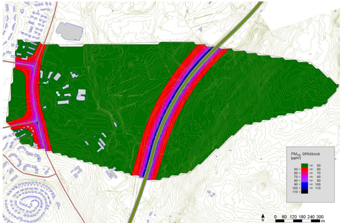
Mynd 11.2: Núverandi ástand. Svífryk PM 10 . Hæsti meðalstyrkur sólarhrings árið 2008 undir 98 % líkindum (7 sólarhringar gætu orðið hærri). Leiðbeinandi heilsuverndarmörk eru 50 µg/m 3 (græn svæði eru undir mörkum).
