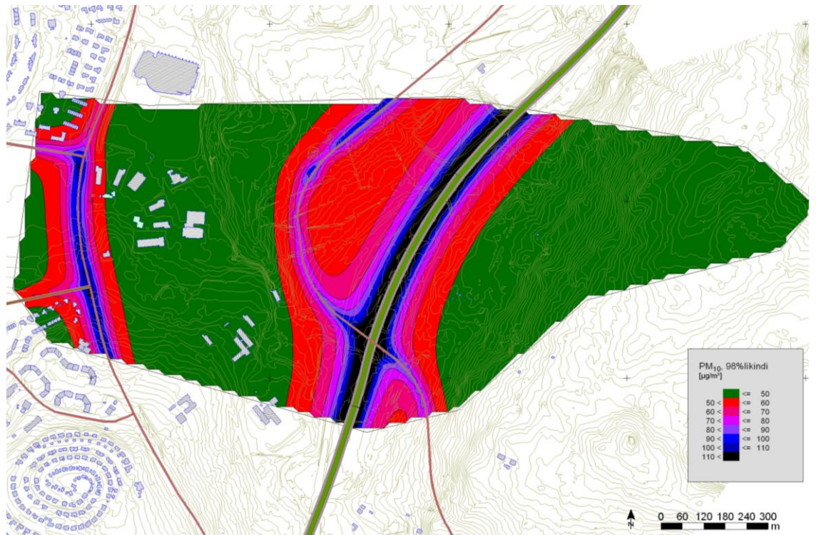
Mynd 11.9: Núllkostur. Svifryk PM 10 . Hæsti meðalstyrkur sólarhrings árið 2024 undir 98 % líkindum (7 sólarhringar gætu orðið hærri). Leiðbeinandi heilsuverndarmörk eru 50 µg/m 3 (græn svæði eru undir mörkum).
